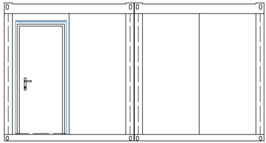
Ansicht C
